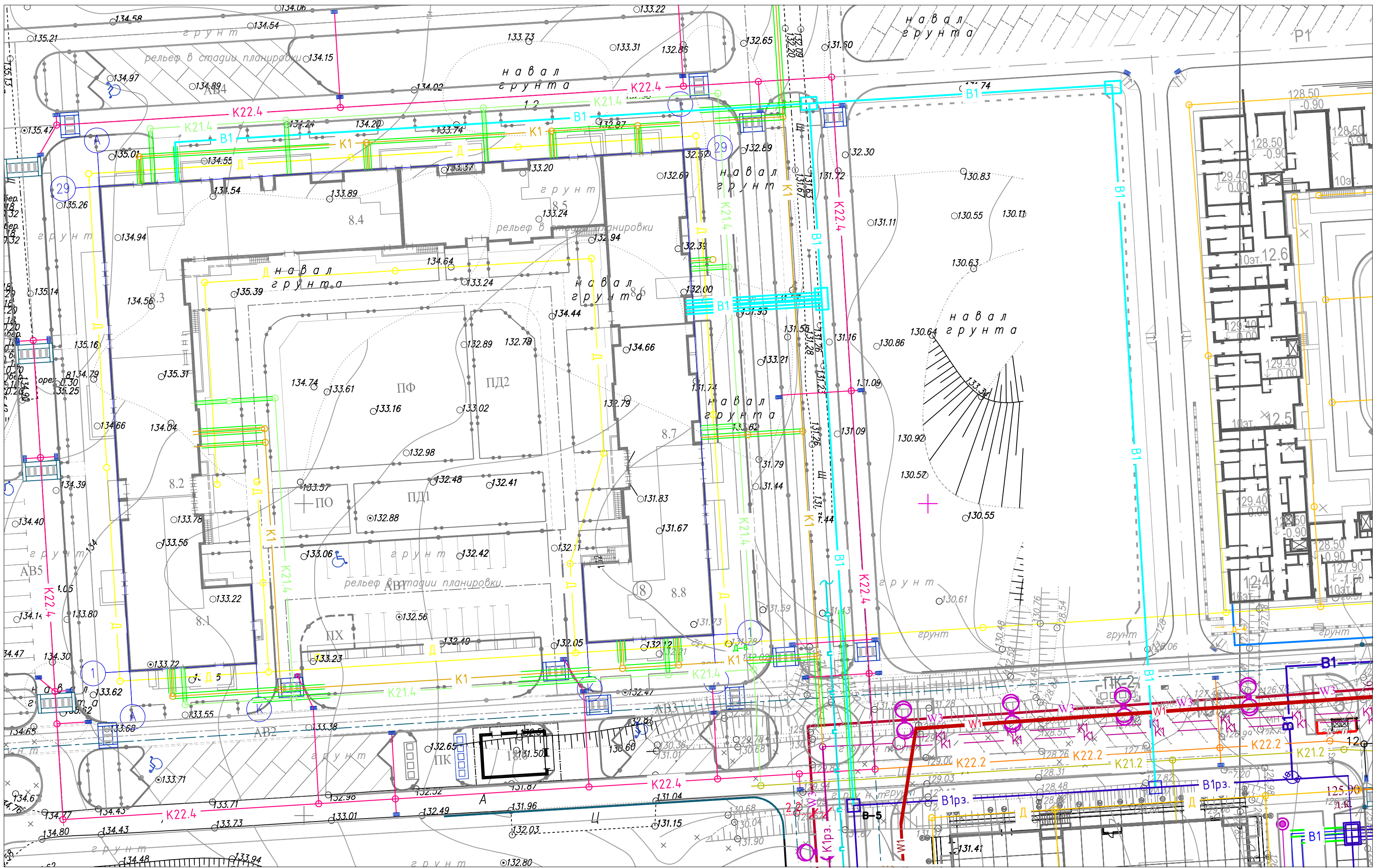
Условные обозначения трубопроводов
